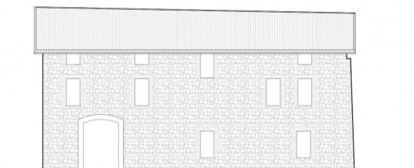
PROSPETTO OVEST
