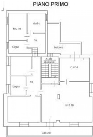
PIANO PRIMO
