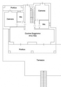
PIANTA PIANO TERRA
