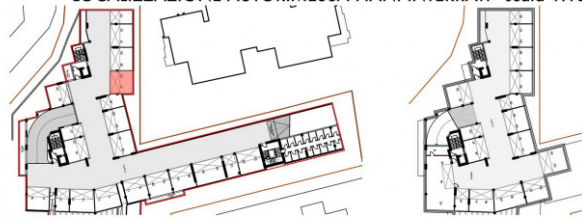
LOCALIZZAZIONE AUTORIZZAZIONE PIANI INTERRATI - scala 1:1000
